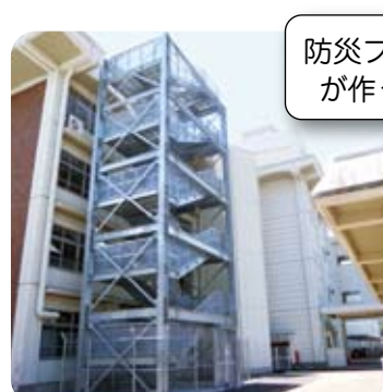
屋上避難用外階段
